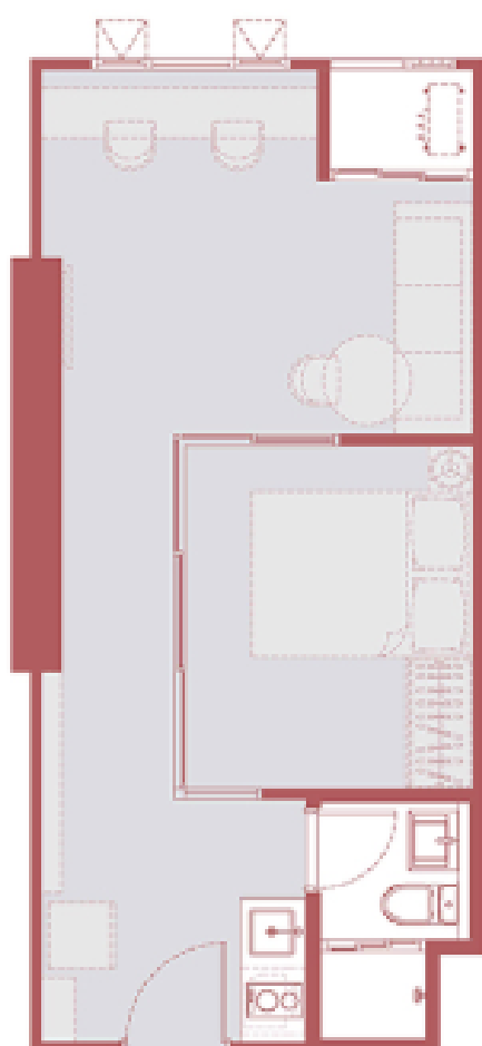
TYPE D1 34.00 SQ.M.
