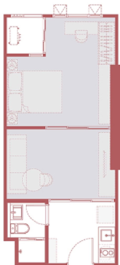
TYPE D2M 34.00 SQ.M.
