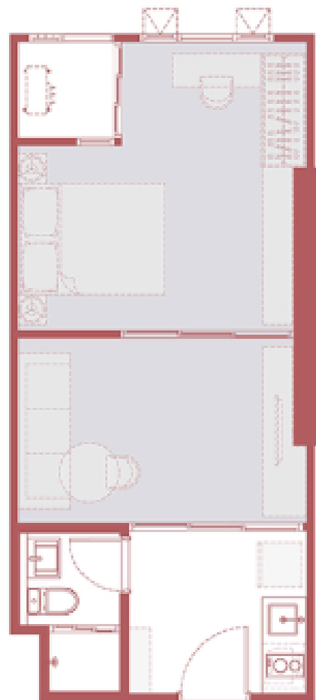
TYPE D2M 34.00 SQ.M.
